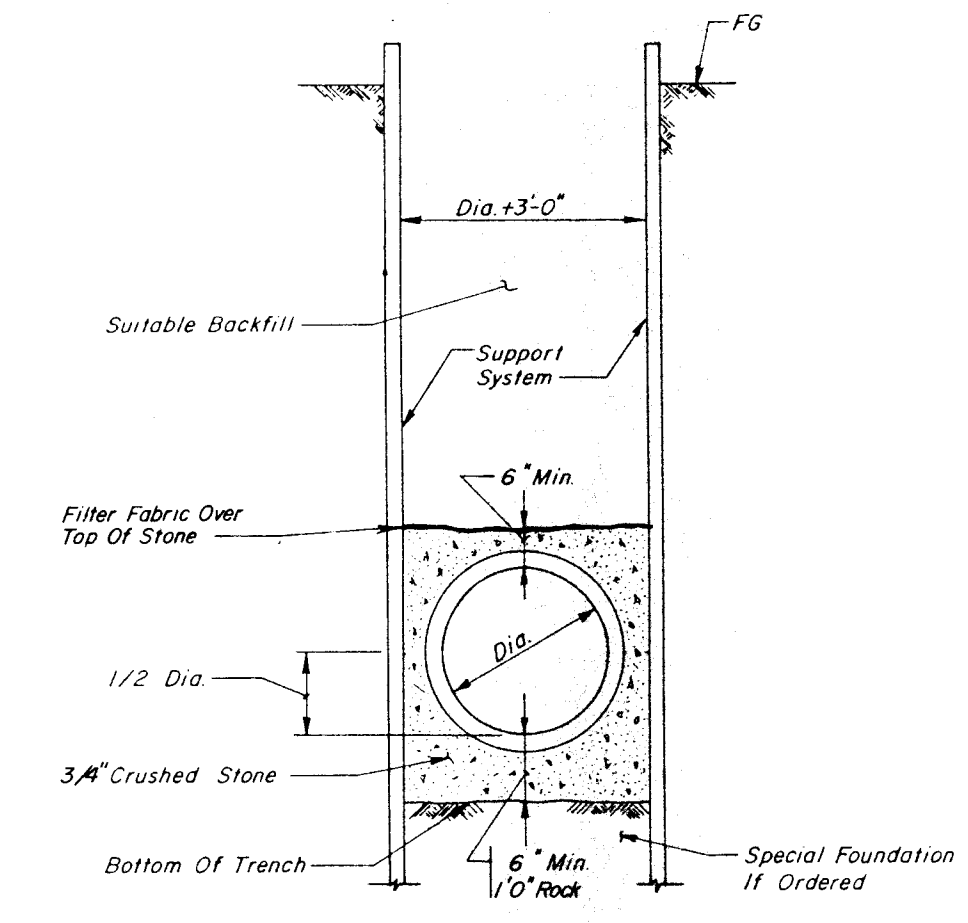
TRENCH DETAIL N.T.S.
